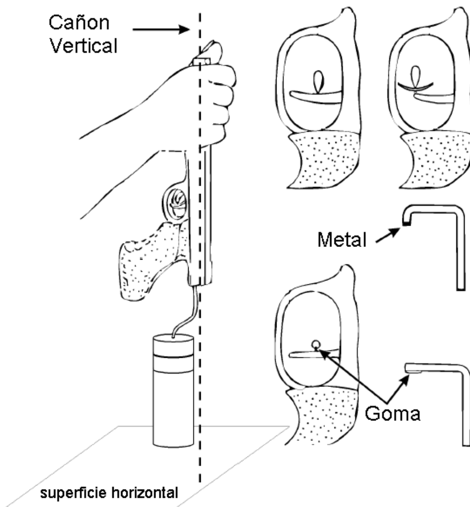
Medida del Peso del Disparador
